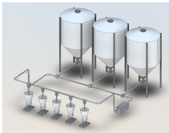
Abb. 23: Grundprinzip einer mehrphasigen Fütterung mit einem Verteilsystem (© KTBL)
