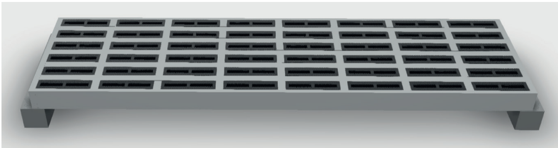
Abb. 14: Perforierter Boden mit Profil und Dichtungsklappen (© KTBL)
