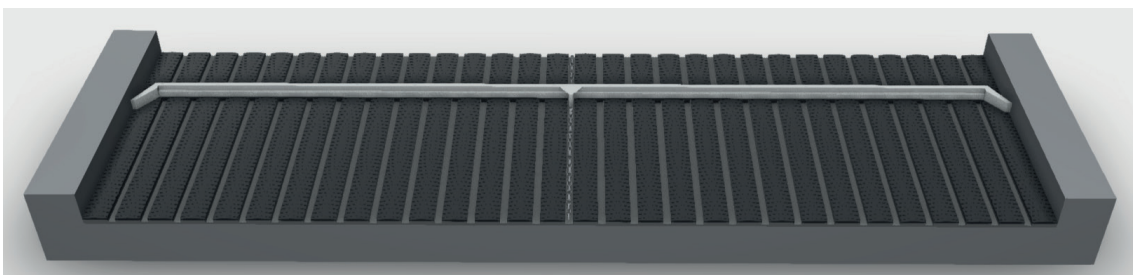
Abb. 22: Planbefestigter Rillenboden mit Profil und Schieber (© KTBL)
