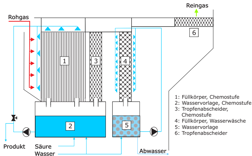
Abb. 3: Prinzip einer zweistufigen Abluftreinigungsanlage (Chemowäsche + Wasserwäsche) (KTBL 2006)
