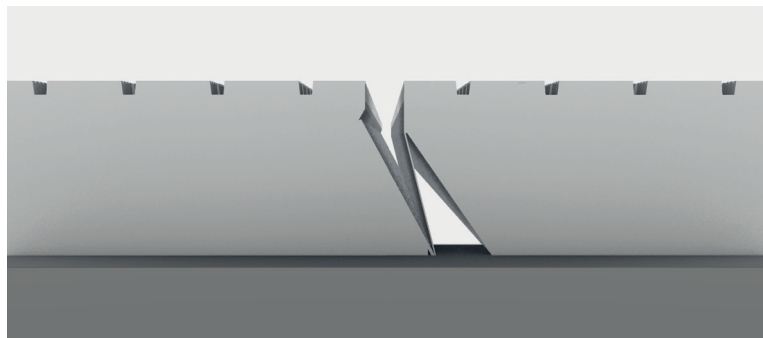
Abb. 11: Bodenelement in seitlicher Ansicht mit Dichtungsklappe im Detail, die den Gasaustausch mit dem Güllekanal reduziert (© KTBL)
