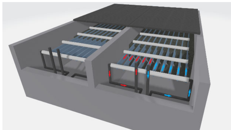
Abb. 27: Güllekühlung mittels Schwimmkühlkörpern (© KTBL)
