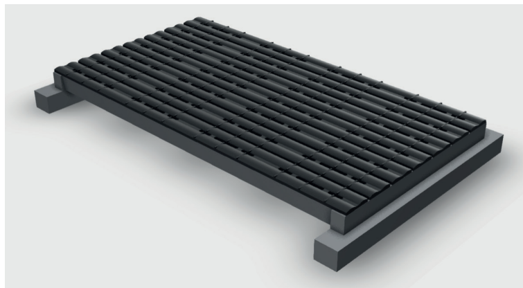
Abb. 18: Gummiauflage mit konvexer Wölbung zum Schlitz; Aufsicht (© KTBL)
