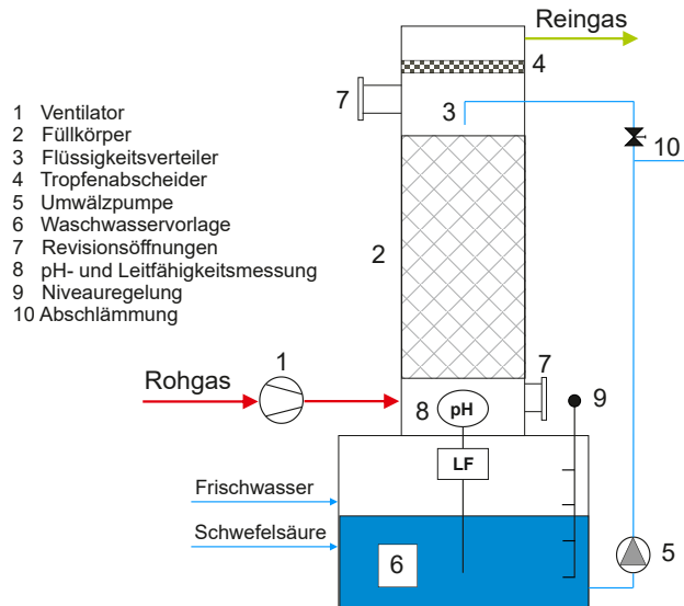
Abb. 2: Grundprinzip eines Rieselbettreaktors (KTBL 2006)
