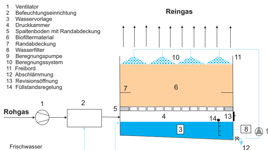
Abb. 1: Grundprinzip eines einstufigen Biofilters (KTBL 2006); hier ohne Ansäuerung
