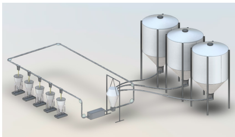
Abb. 25: Grundprinzip einer Multiphasenfütterung mit einem Chargenmischer und Verteilung über ein Verteilsystem (© KTBL)
