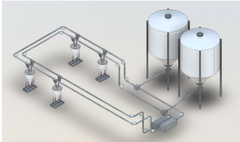
Abb. 24: Grundprinzip einer 2-phasigen Fütterung mit zwei parallel angeordneten Verteilsystemen (© KTBL)
