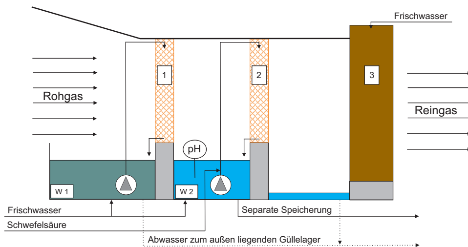
Abb. 3: Prinzip einer zweistufigen Abluftreinigungsanlage (Chemowäsche + Wasserwäsche) (KTBL 2006)
