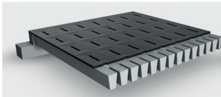
Abb. 16: Auf Spaltenbodenelementen verlegte Gummimatte mit reduziertem Schlitzanteil (© KTBL)
