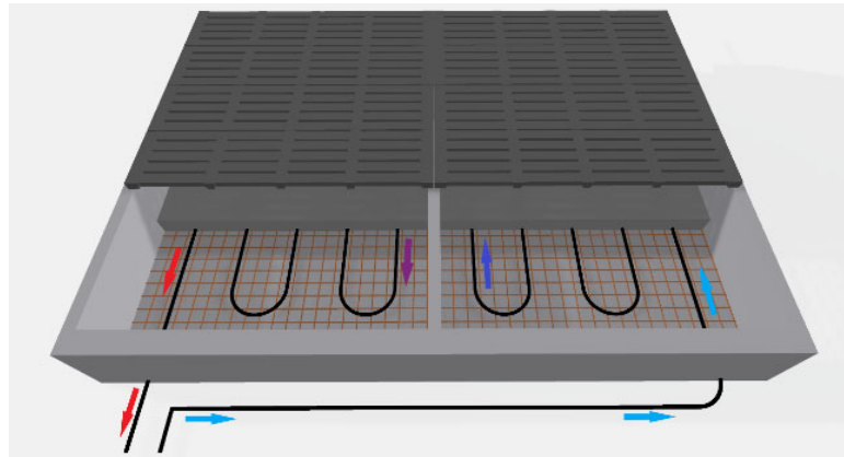
Abb. 26: Güllekühlung mittels im Boden verlegten, auf der Bewehrung aufliegenden Kühlleitungen (© KTBL)
