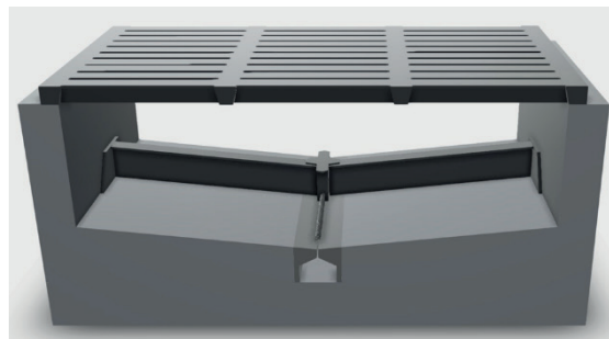
Abb. 5: Unterflurschieber mit Kot-Harn-Trennung in der Mastschweinehaltung (© KTBL)
